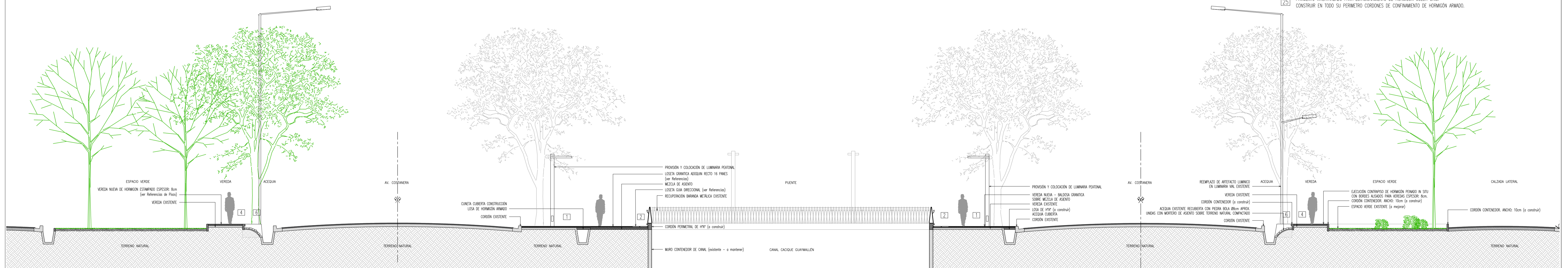
PERFIL CRUCE CALLES LAVALLE - GODOY CRUZ
