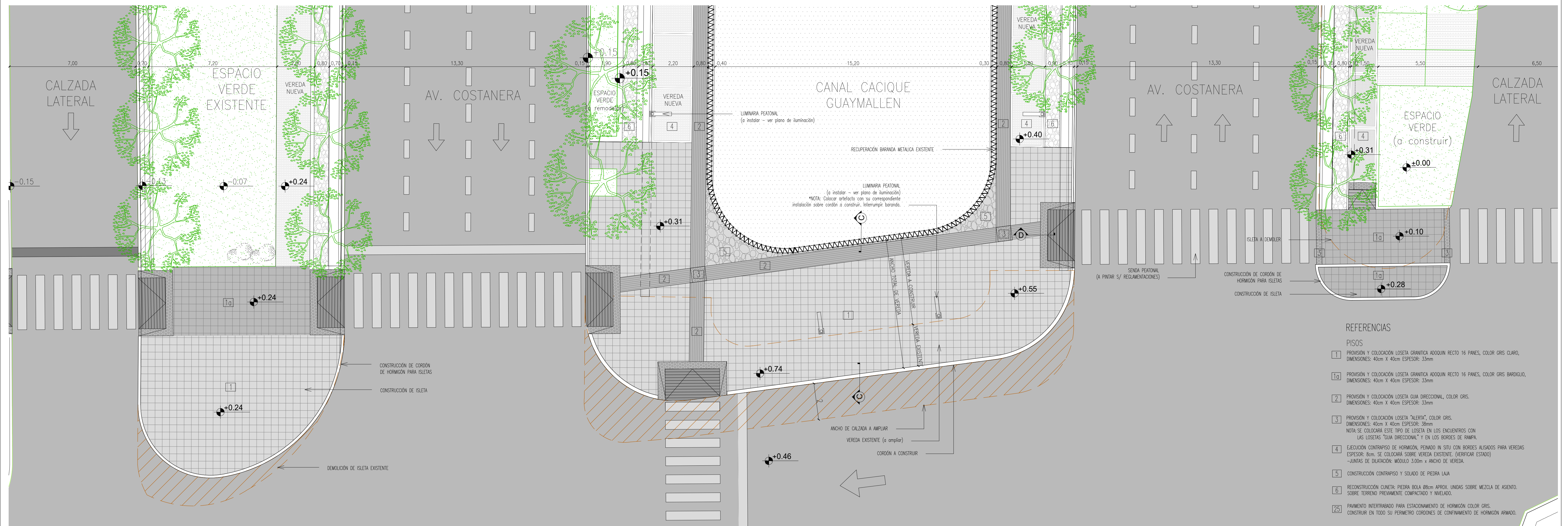
PLANTA CRUCE CALLES CATAMARCA - TOSO
