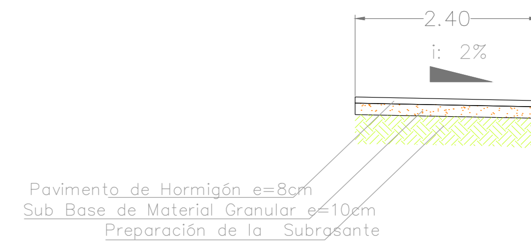
Detalle Constructivo Ciclovia Oeste Esc. 1:50
