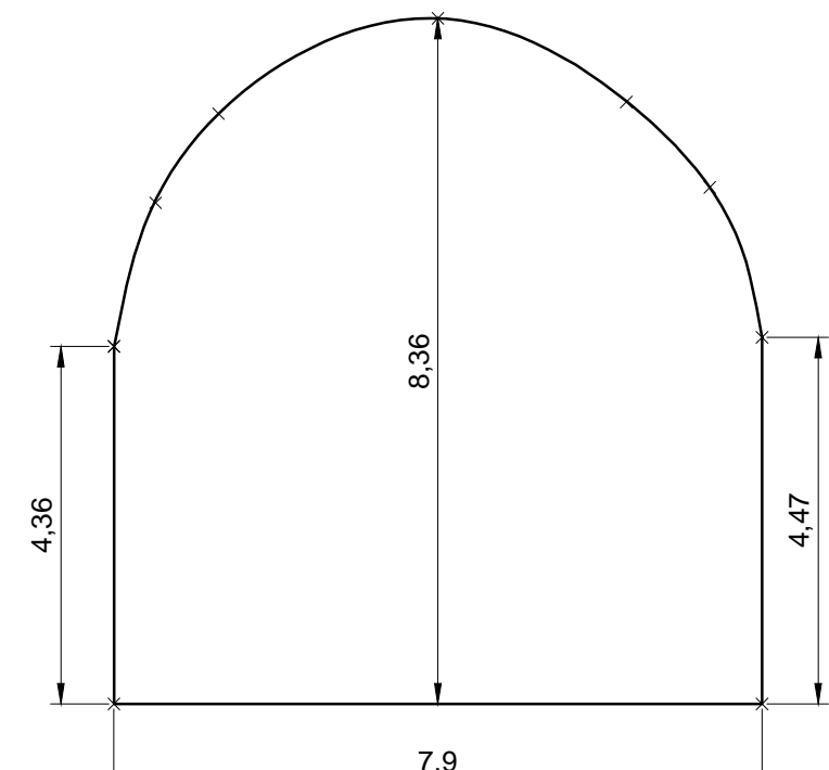
Perfil transversal 3 prog. 165.00- Long bóveda: 12.15m
