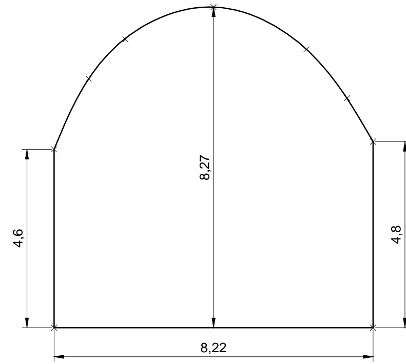
Perfil transversal 4 prog. 215.00- Long Bóveda. 11.55m
