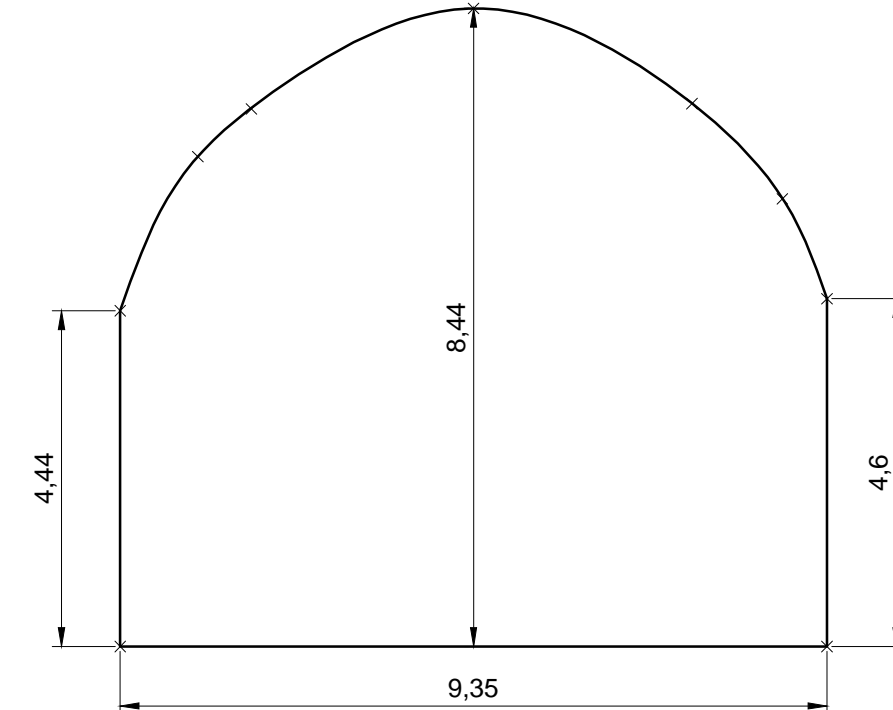
Perfil transversal 5 prog. 265.00- Long Bóveda. 12.95m
