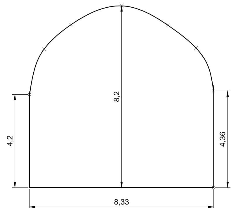
Perfil transversal 2 prog. 115.00- long Bóveda: 12.40m
