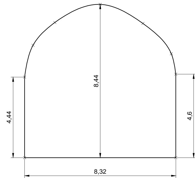
Perfil transversal 1 prog. 65.00- Long Bóveda: 12.40m
